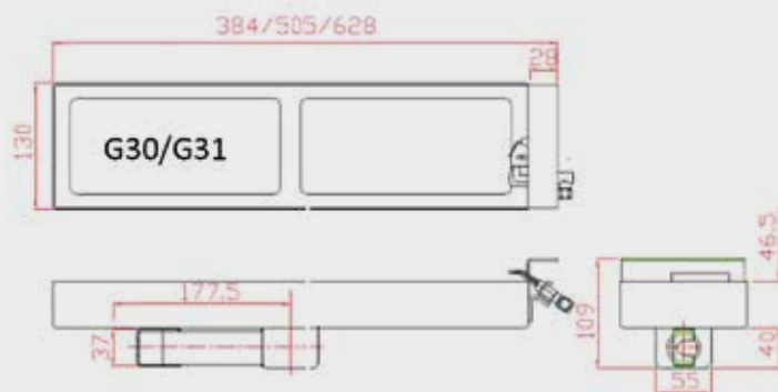
Brûleur Butane/Propane G30/G31
